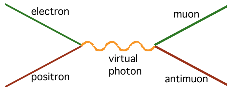
Feynman diagram
